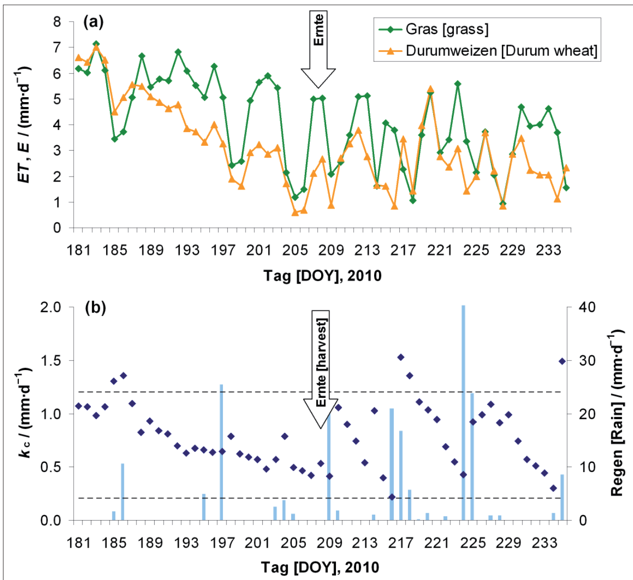
Abbildung 3: Verdunstung von Gras und Durum am Lysimeter gegen Ende der Vegetationsperiode und danach (Ernte am 28.7.2010 / Tag 208); die gestrichelten Linien repräsentieren den k_{c,b} Wert (untere) bzw. den maximalen k_{c,b} Wert (obere)
