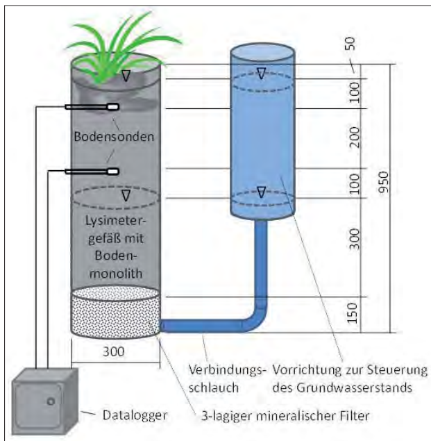
Abbildung 2: Prinzipskizze des Kleinlysimeters
