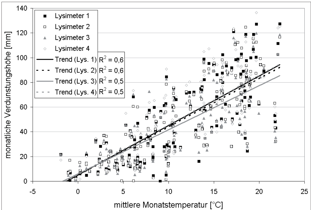
Abbildung 9: Korrelation der monatlichen Verdunstungshöhen mit der mittleren monatlichen Temperatur an der Messtation Niederwerth
