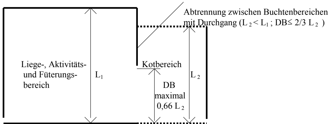
Abbildung 2: Erläuterung der höchstmöglichen Durchgangsbreite DB in „Abtrennungen zwischen Buchtenbereichen“ gemäß Fußnote 3) zu Spalte f der Tabelle 4
