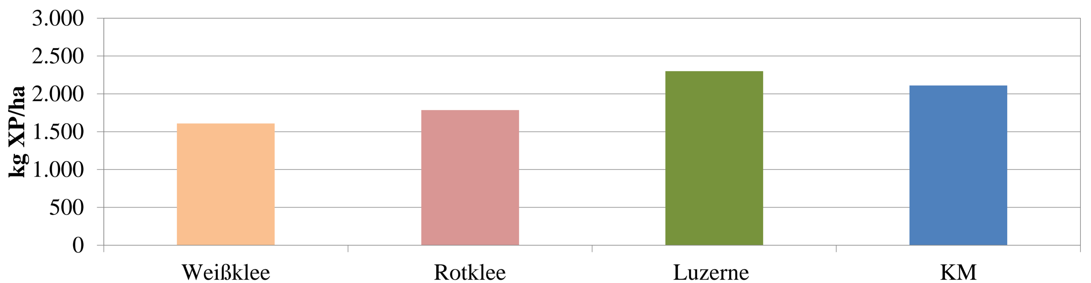
XP-Ertrag 2008
