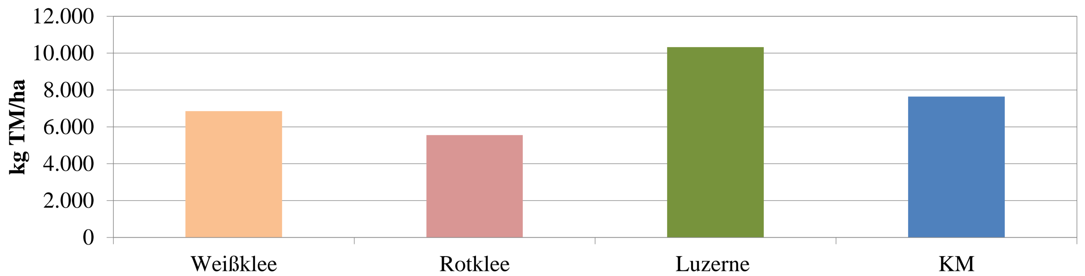
TM-Ertrag 2009
