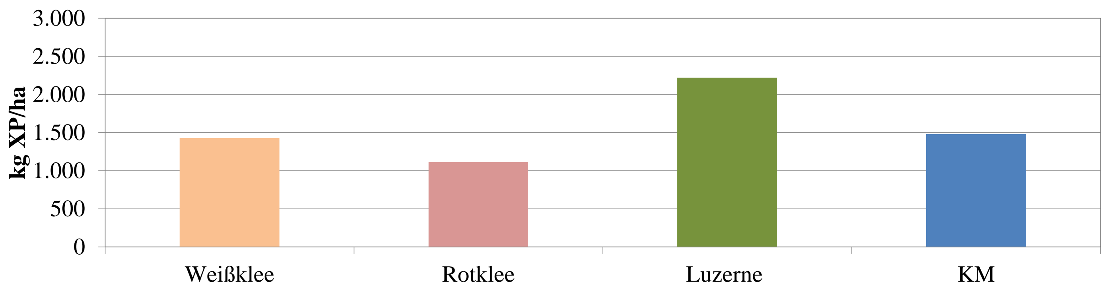
XP-Ertrag 2009
