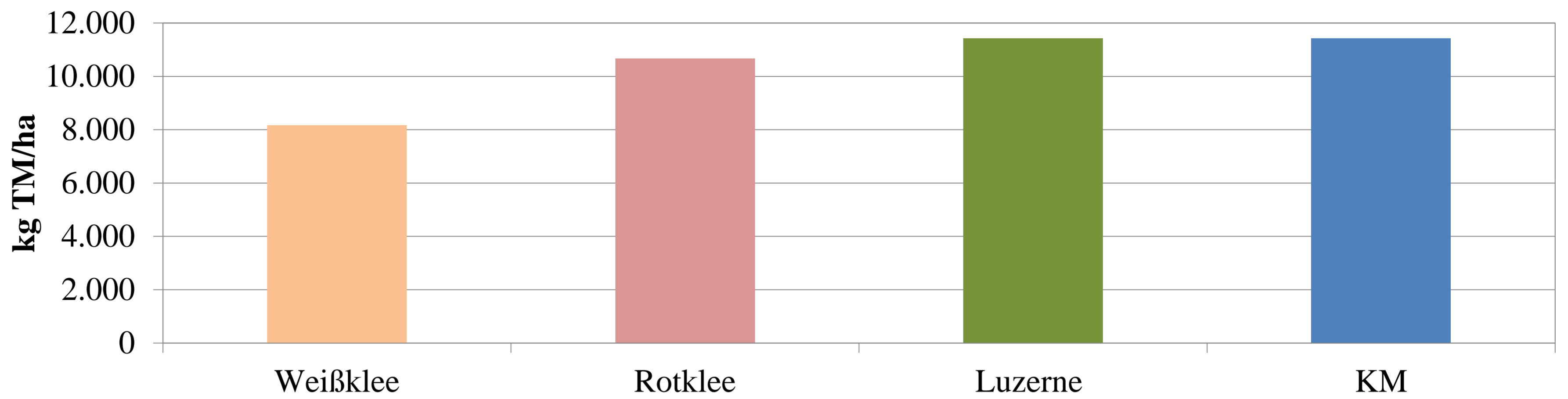
TM-Ertrag 2009
