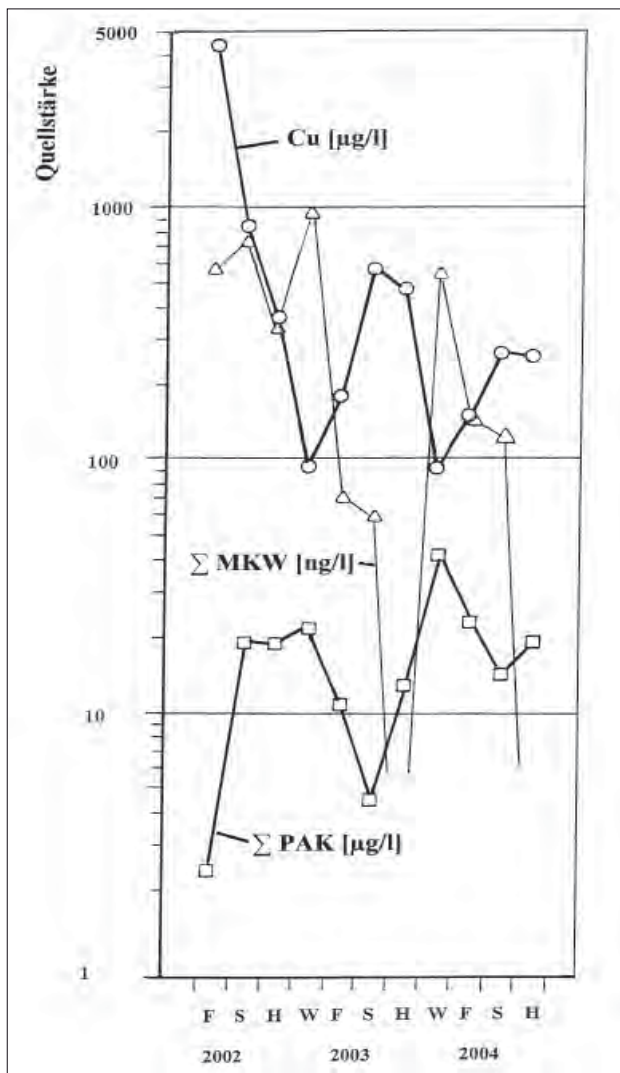
Abbildung 3: Zeitlicher Verlauf der Cu- (Messpunkte: ○), der PAK- (□) und der MKW-Quellstärke (Δ) aus den Altlastensylometern MV, BS bzw. BO während der Betriebszeit 02/2002 bis 11/2004.
