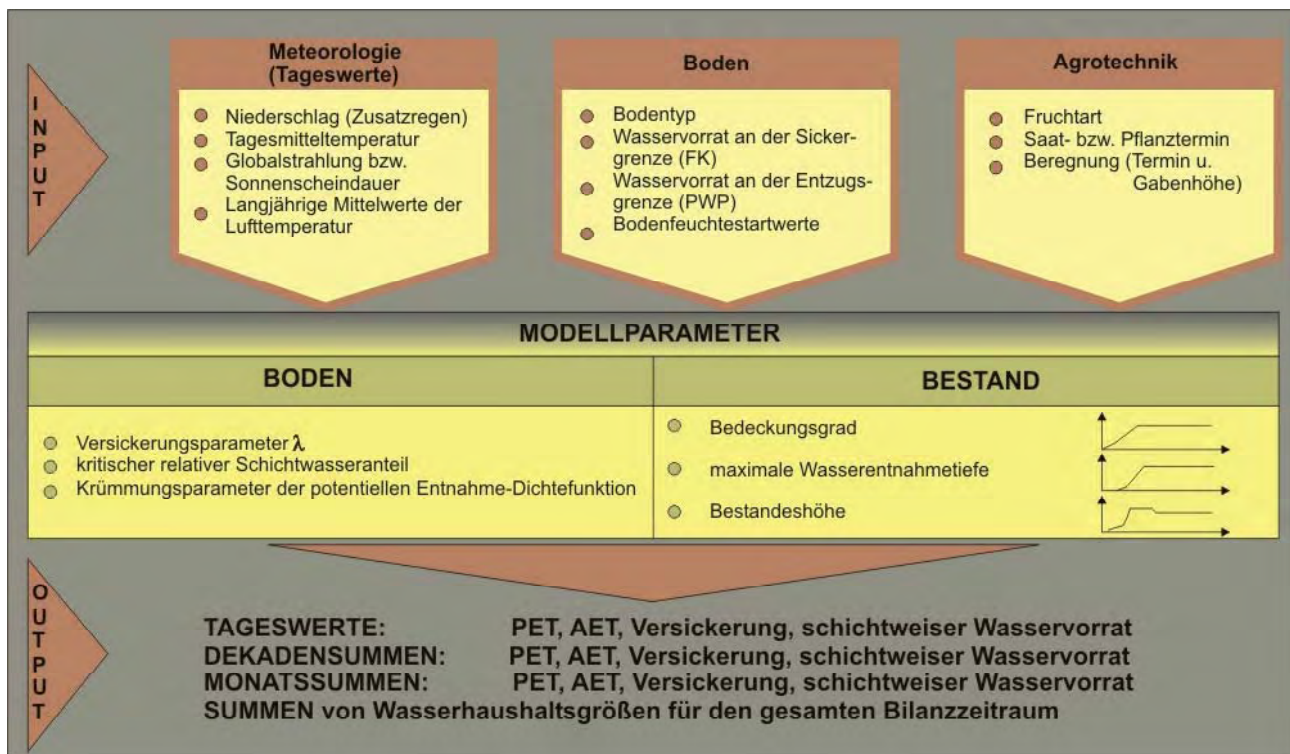
Abbildung 4: Input- und Outputparameter des Mehrschichtenbodenfeuchte- und Evapotranspirationsmodells BEREST (WENKEL et al. 2006)
