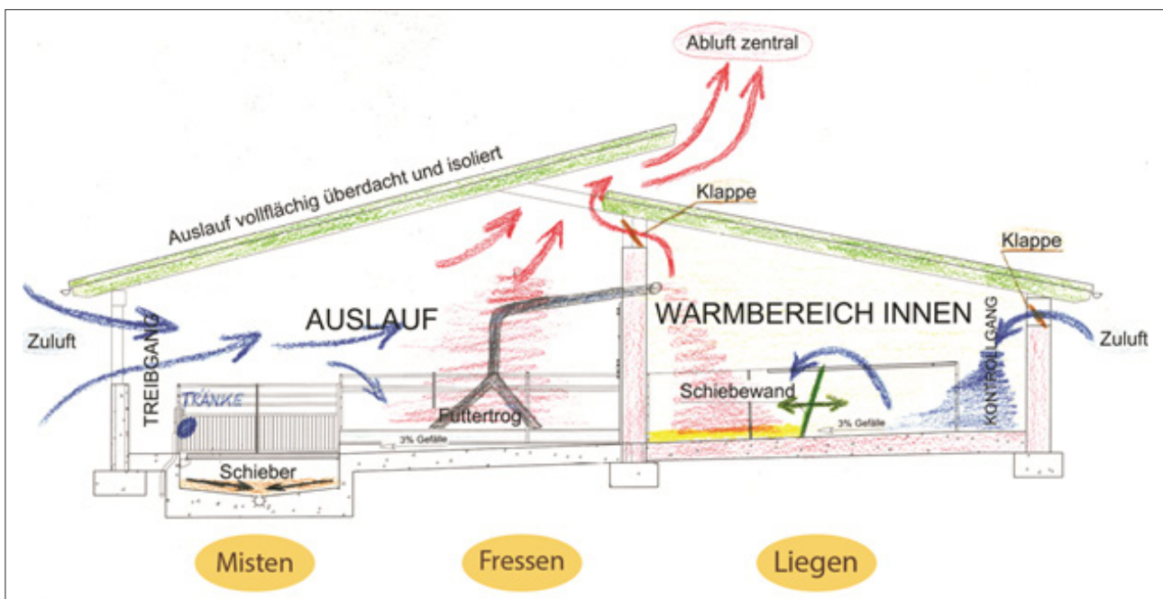
Abbildung 4: Querschnitt des emissionsarmen Tierwohlmaststalls mit Darstellung der Funktionsbereiche und Luftführung (Quelle: Schauer Agrotronic GmbH)
