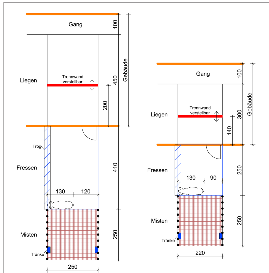
Abbildung 8: Buchtenkonzept für 25 Mastschweine (links) und 15 Tiere (rechts)
