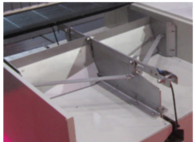
Abbildung 7: Schieberentmistungstechnik im Auslaufbereich (Quelle: Schauer Agrotronic GmbH)
