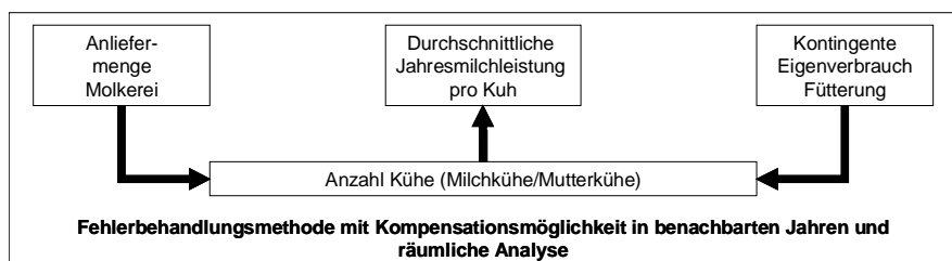
Abbildung 2: Datenschema Milchleistung
