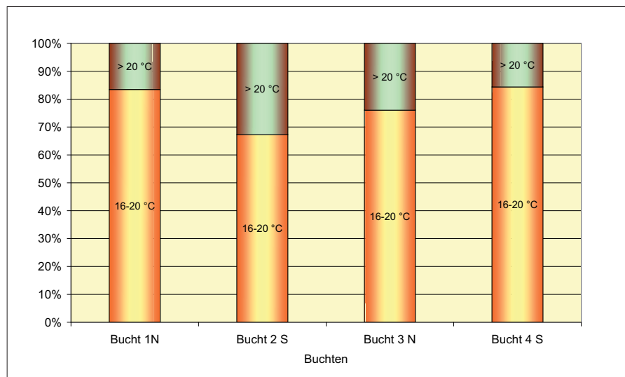
Abbildung 8: Temperaturverteilung Winterdurchgang
