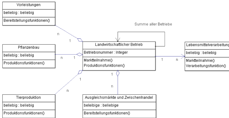
Abbildung 4: UML-Diagramm der inländischen Nahrungsbereitstellung
