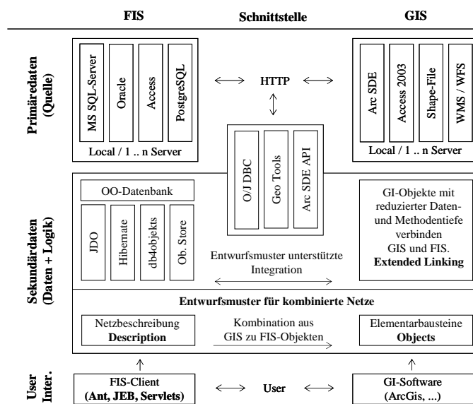
Abbildung 1: Systementwurf der Agricultural-GIS-Sphere
