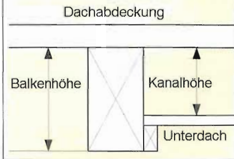
Abb. 14: Die Kollektorkanäle bestehen in der Regel aus den Balken (Pfetten oder Sparren), der Dachabdeckung und der Luftleitplatte (Unterdach). Die optimale Kanalhöhe wird ausgehend von der maximalen Balkenhöhe berechnet.
