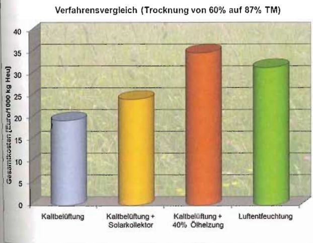
Abb. 21: Gesamtkosten je 1.000 kg Heu bei Trocknung von 60 % auf 87 % TM (Preisbasis Jänner 2009, Stromtarif 13 Cent/kWh, Ölpreis 0,6 Euro/l, ohne Kosten der Heuwerbung und ohne Gebäudekosten).
