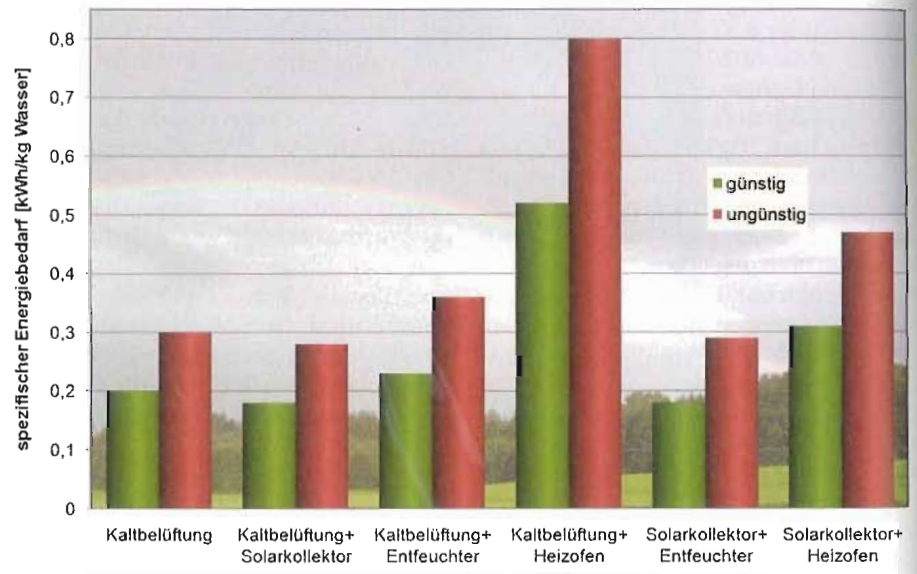
Abb. 20: Spezifischer Energiebedarf verschiedener Verfahren
