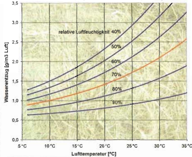
Abb. 5: Maximaler Wasserentzug in g/m³ Luft bei 60 % TM
