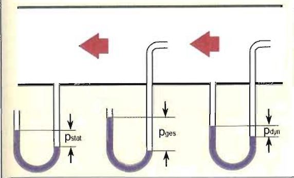
Abb. 9: Druckmessung, links statischer Druck, Mitte Gesamtdruck, rechts dynamischer Druck
