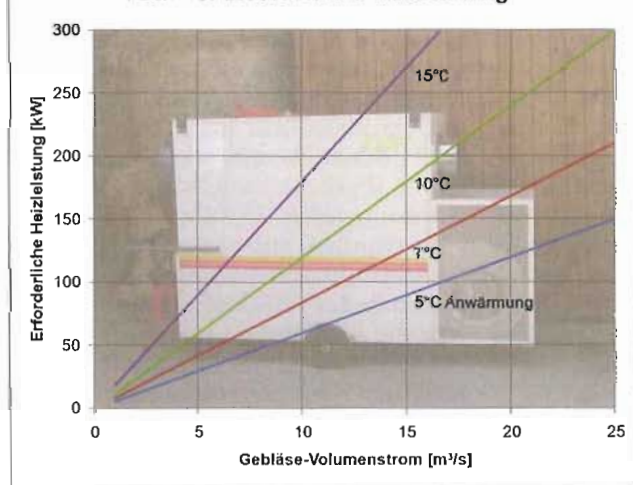
Abb. 10: Erforderliche Heizleistung
