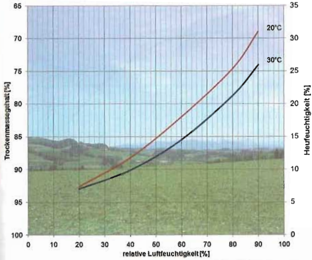
Abb. 3: Feuchtigkeitsgleichgewicht von Wiesenheu (nach Segler, 1968)
