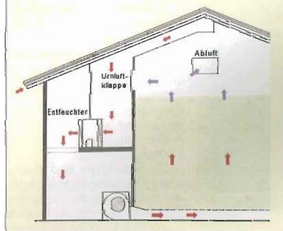
Abb. 17: Anlagenschema mit Luftentfeuchter und Dachabsaugung (Variante Entfeuchtung im Hauptstrom)
