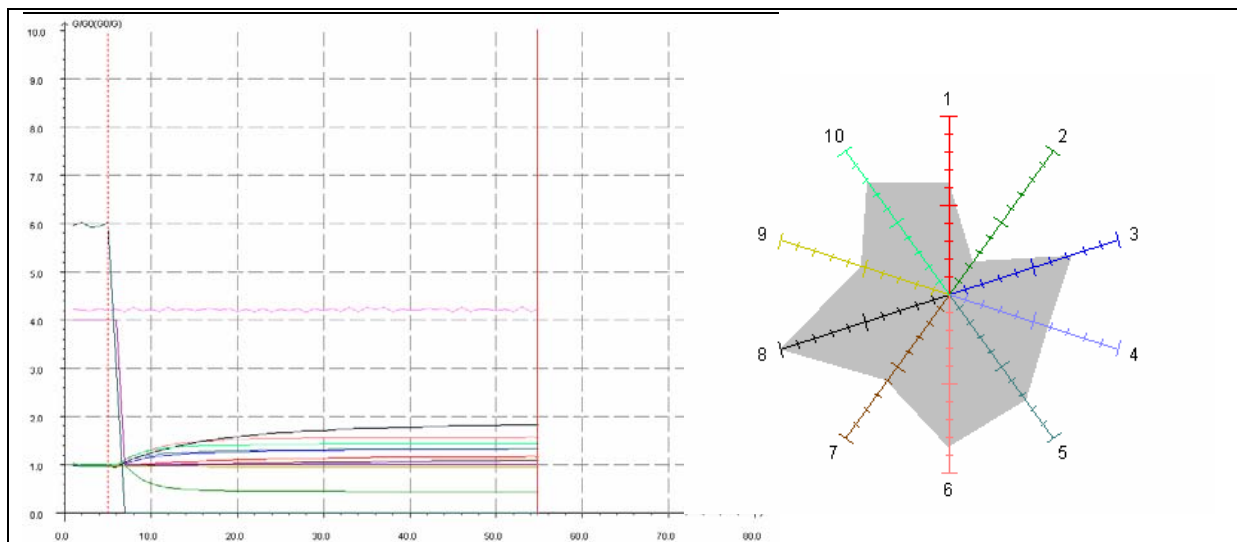
Abbildung 21: Messdatei Kontrolle
