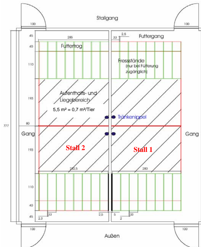
Abbildung 2: Planskizze Aufstallung
