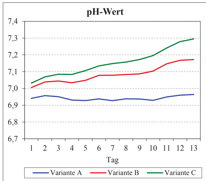
Abbildung: Einfluss der drei Rührvarianten (A) nicht gerührt, (B) einmal pro Tag 60 min gerührt und (C) 6-mal pro Tag 10 min gerührt auf den pH-Wert von Rindergülle
